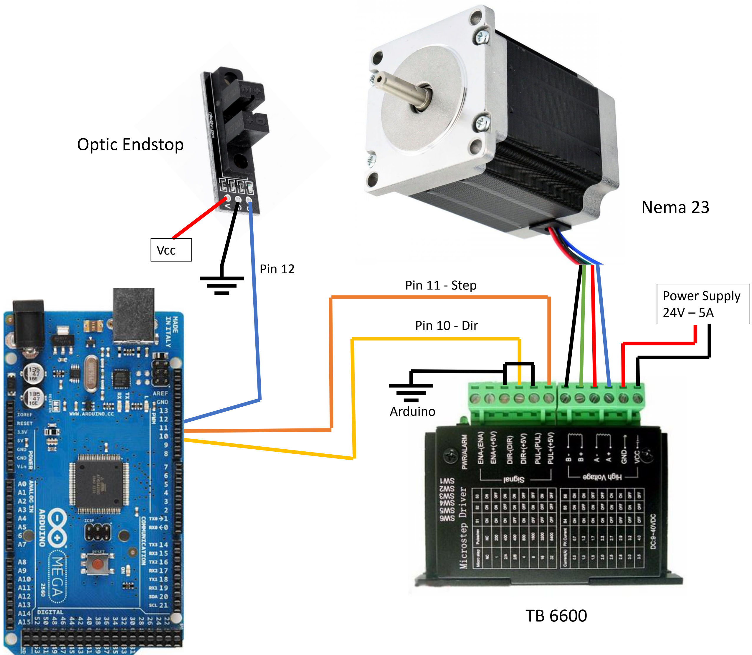
Arduino Mega
